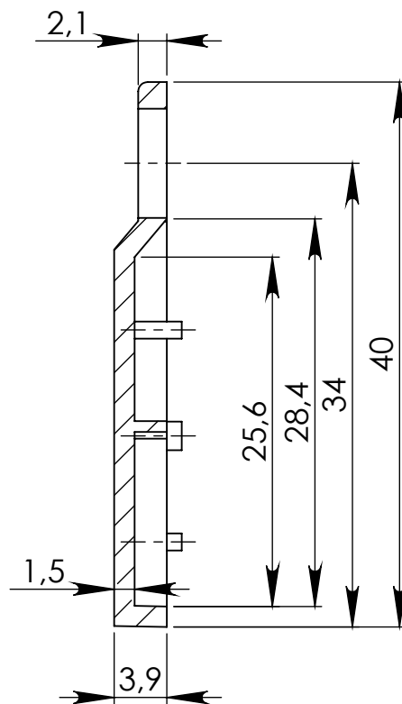
PRZEKRÓJ A-A
